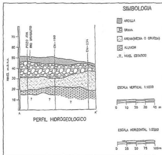
Perfil Hidrogeológico
