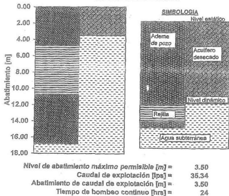
Fig 6 - Indica un perfil del armado del pozo de bombeo, con su ademe y rejilla. Además se indica el caudal y abatimiento de explotación; así como, el tiempo de bombeo continuo recomendado.
