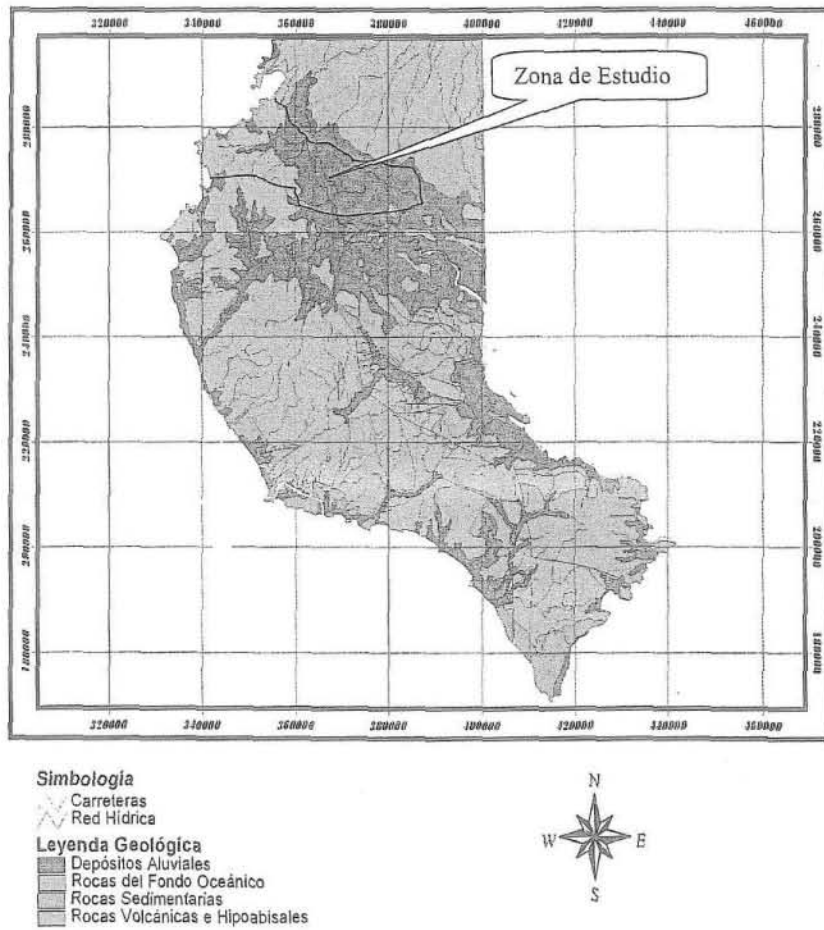
Fig. 2 Mapa Geológico
