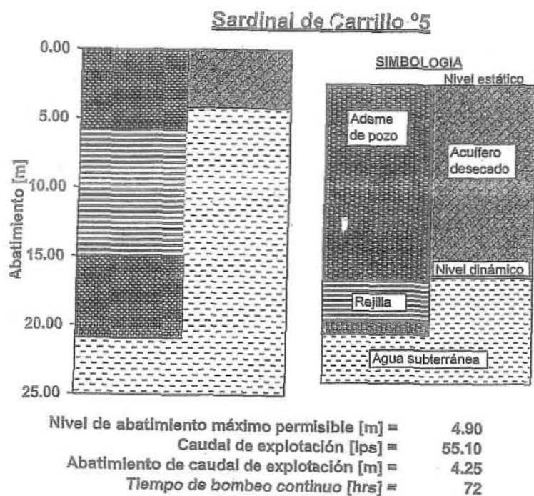
Fig5 - Indica un perfil del armado del pozo de bombeo, con su ademe y rejilla. Además se indica el caudal y abatimiento de explotación; así como, el tiempo de bombeo continuo recomendado.
